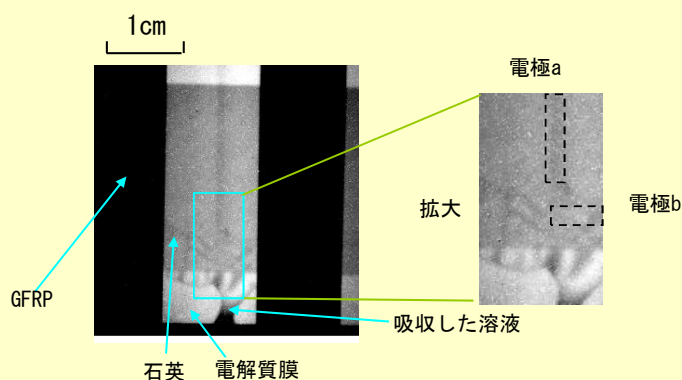
図4 溶液を吸収した電解質膜のラジオグラフィ像
