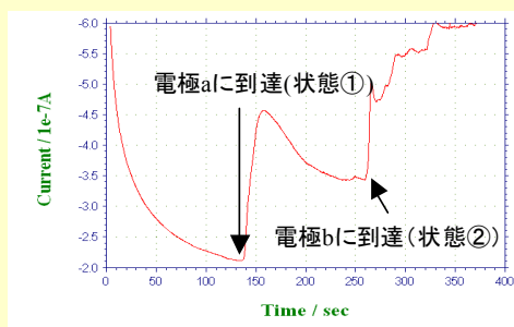
図3 電極a-b間の電流値と時間の関係
