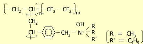
図1 グラフト重合膜の分子構造
