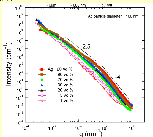
図1 Ag/ワックス微粒子混合試料におけるSANSおよびUSANS実験結果。
