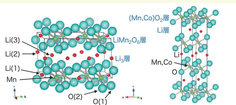
図2 \text{Li}_2\text{MnO}_3 型構造
